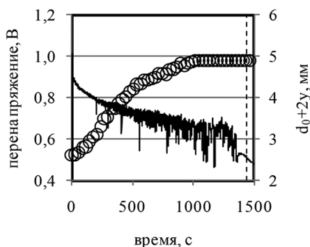
Рис. 2. Динамика изменения диаметра электрода с осадком (O) и катодного перенапряжения (линия) в ходе одноимпульсного электролиза
