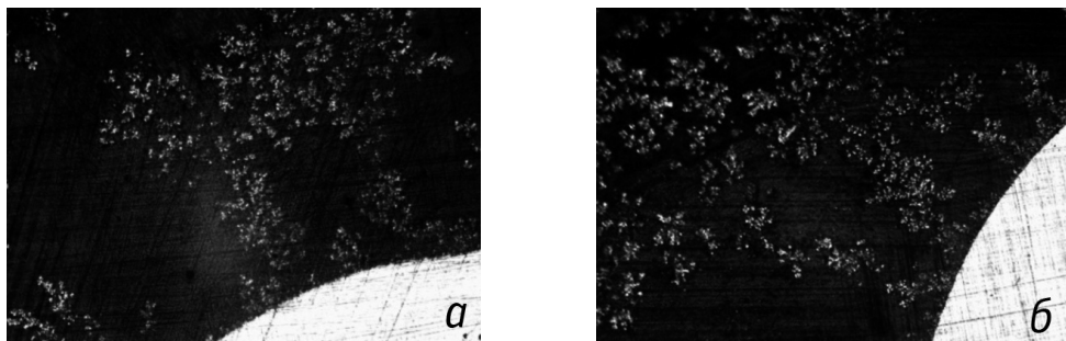
Рис. 7. Микрофотографии поперечного среза электрода с дендритным осадком. Время электролиза, мин.: а – 18; б – 19,5. Увеличение \times 10
